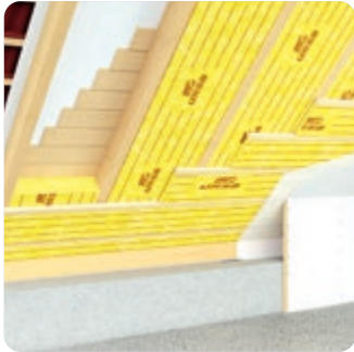
Zwischen- und Untersparrendämmung
